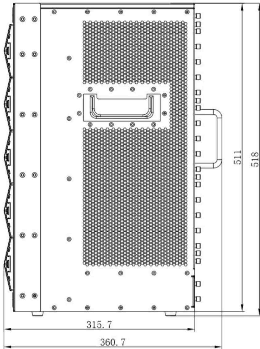
侧面尺寸图
