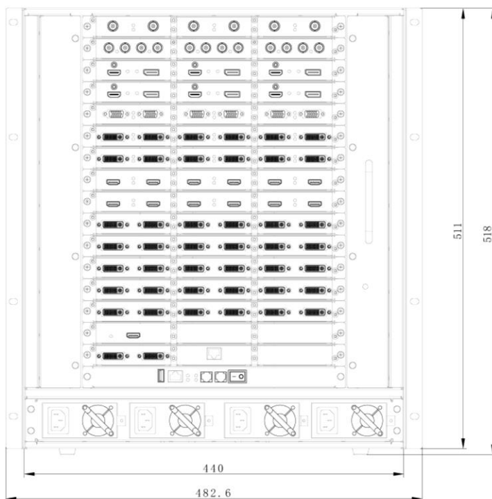
后面板尺寸图
