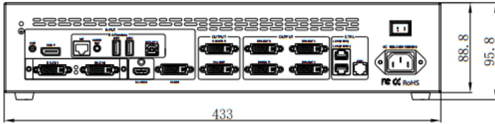
后面板尺寸图
