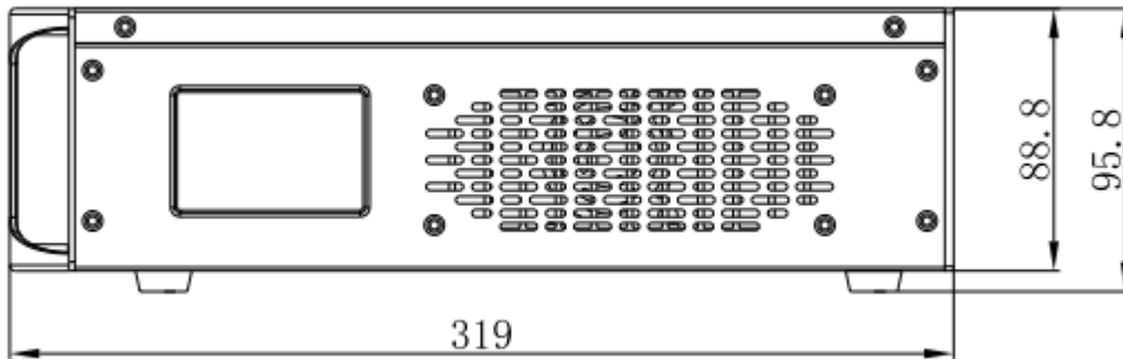
侧面尺寸图
