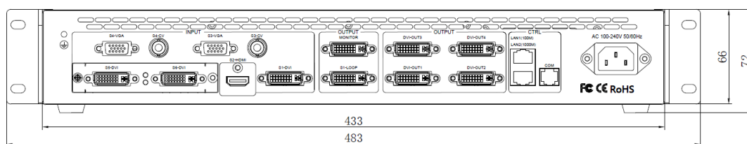
后面板尺寸图
