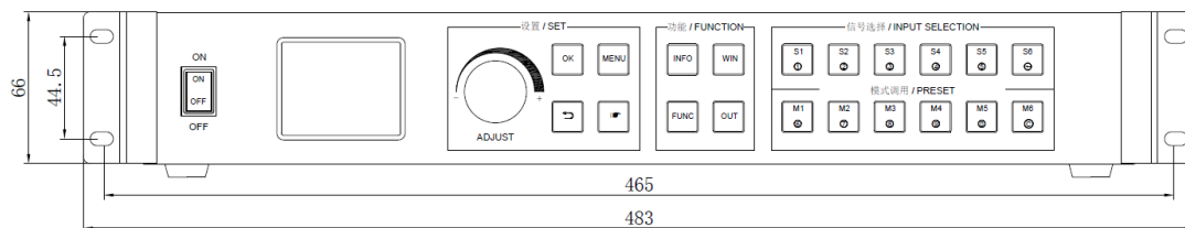
前面板尺寸图
