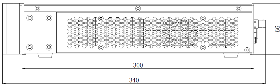
侧面尺寸图
