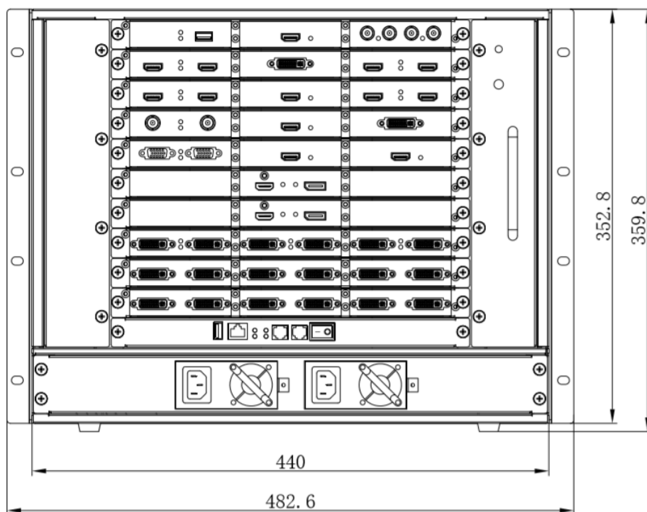
后面板尺寸图
