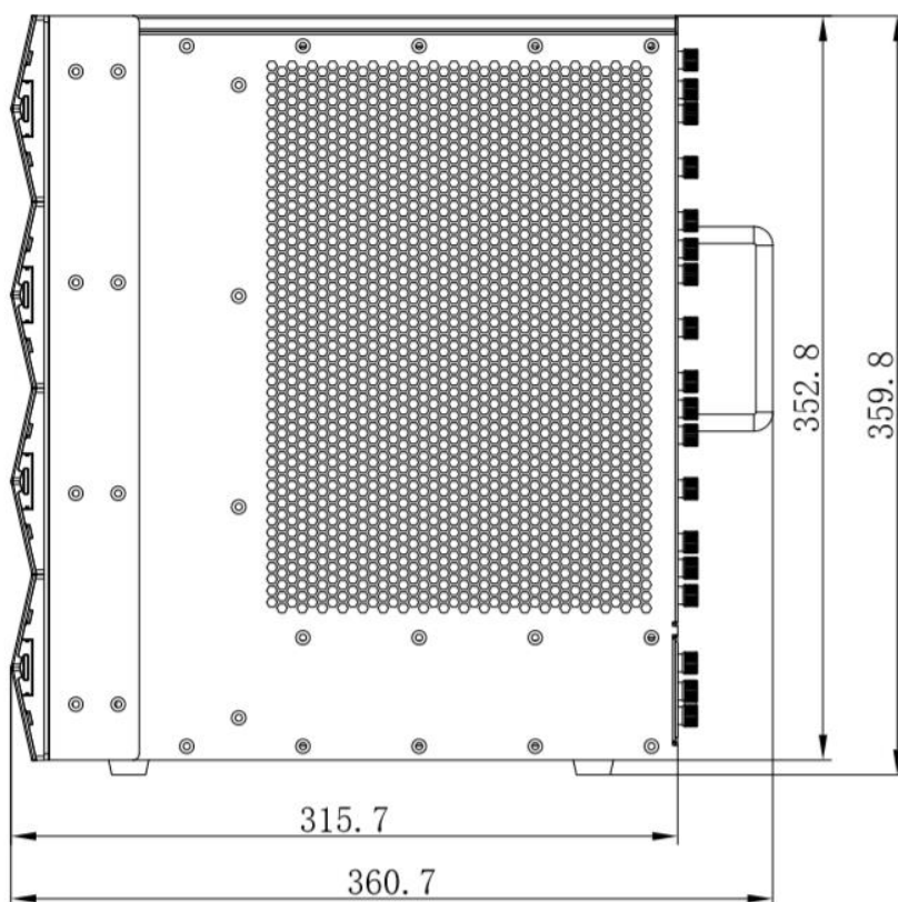
侧面尺寸图
