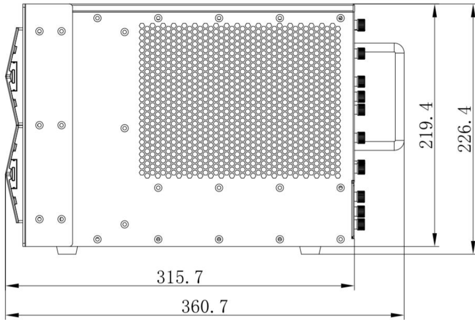
侧面尺寸图
